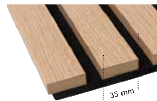
UNIKA 35 Lamelbredder: 35 mm
